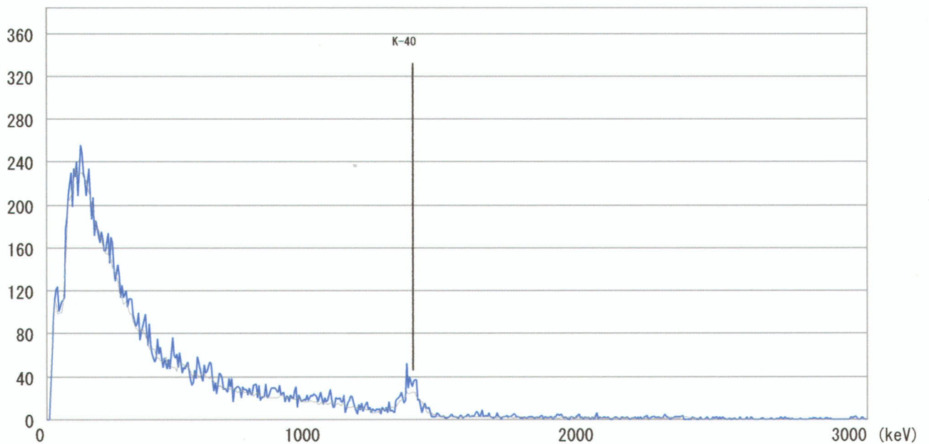
スペクトル解析結果 (データID: 804)
