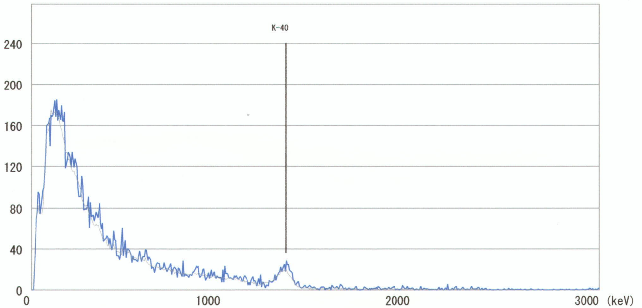
スペクトル解析結果 (データID: 1243)
